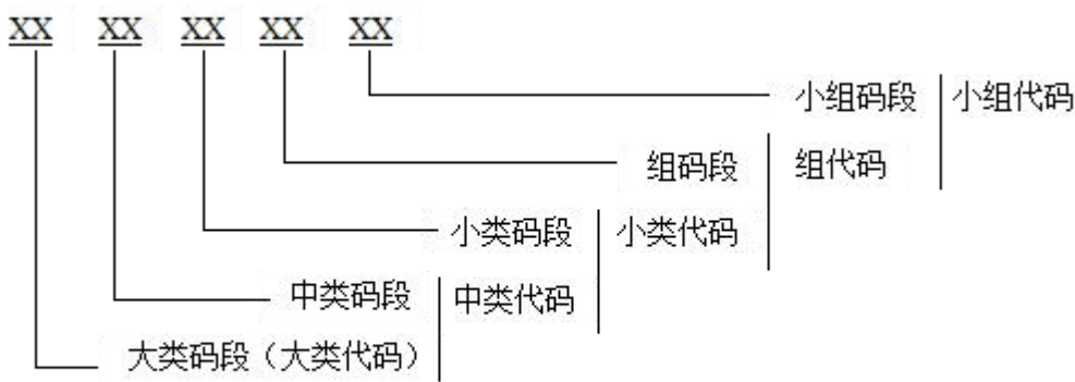
图 1 代码结构
