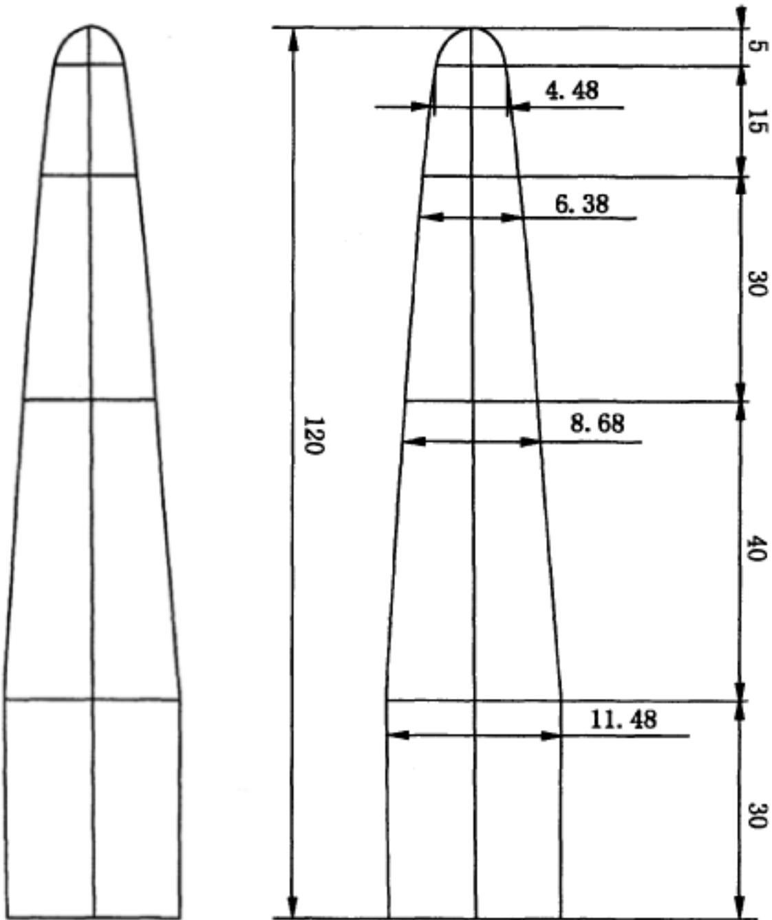
图 D.1 公貂植板示意图
