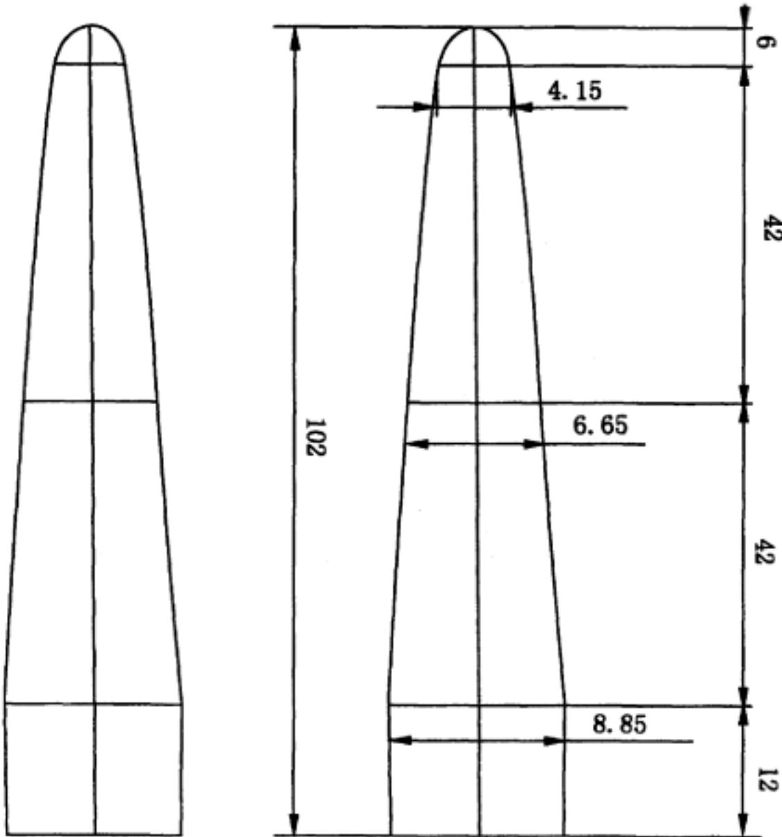
图 D.2 母貂植板示意图
