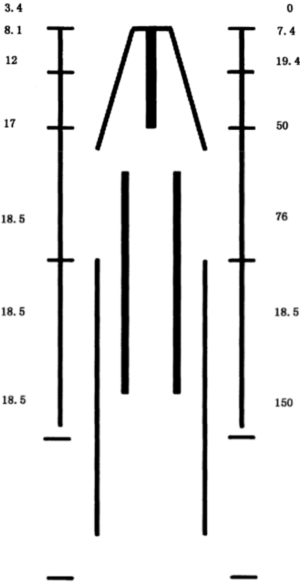
图 D.3 狐、貉植板示意图
