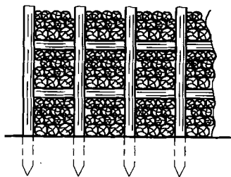
图 8 方格捆楞
