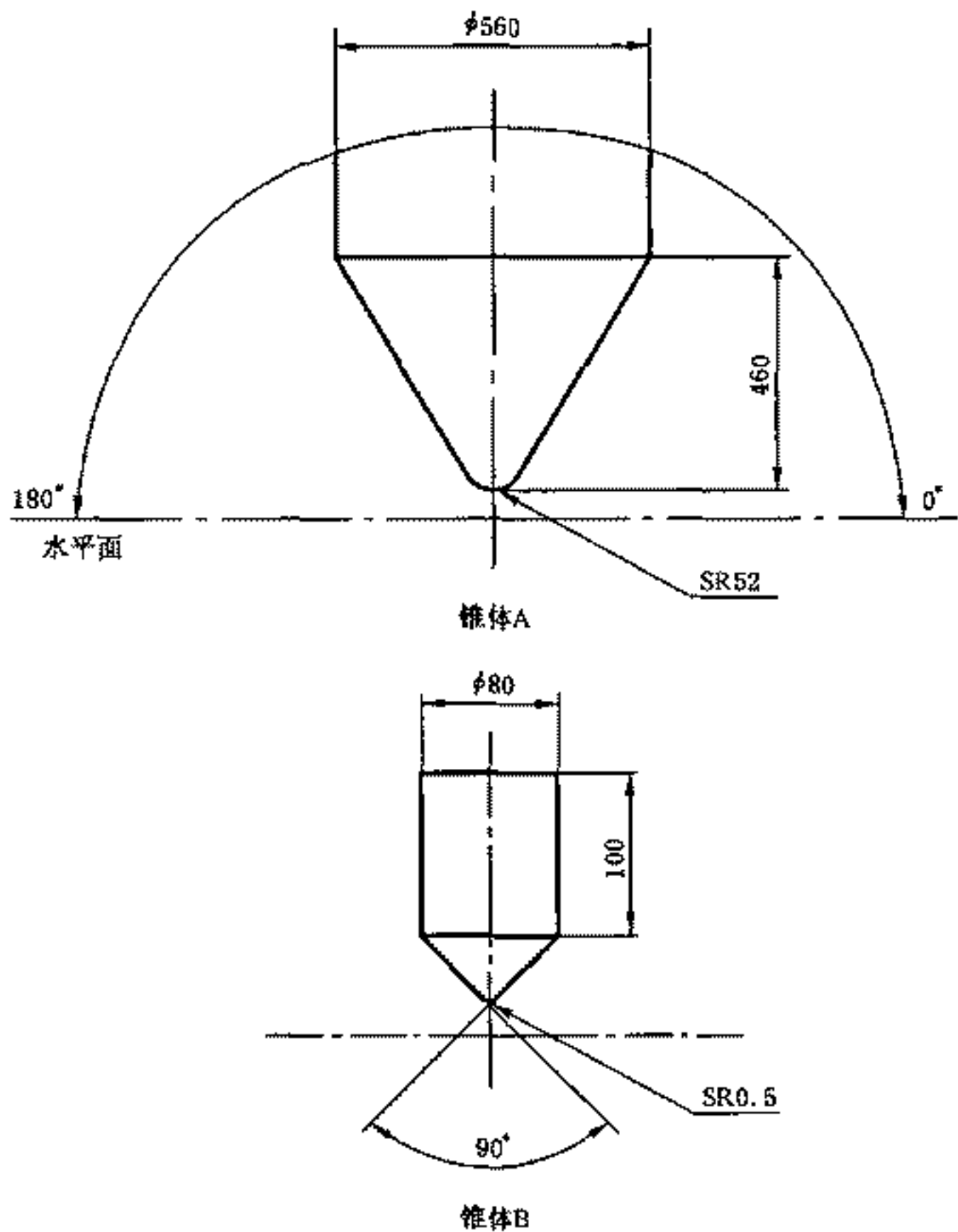
图 2 试验锥
