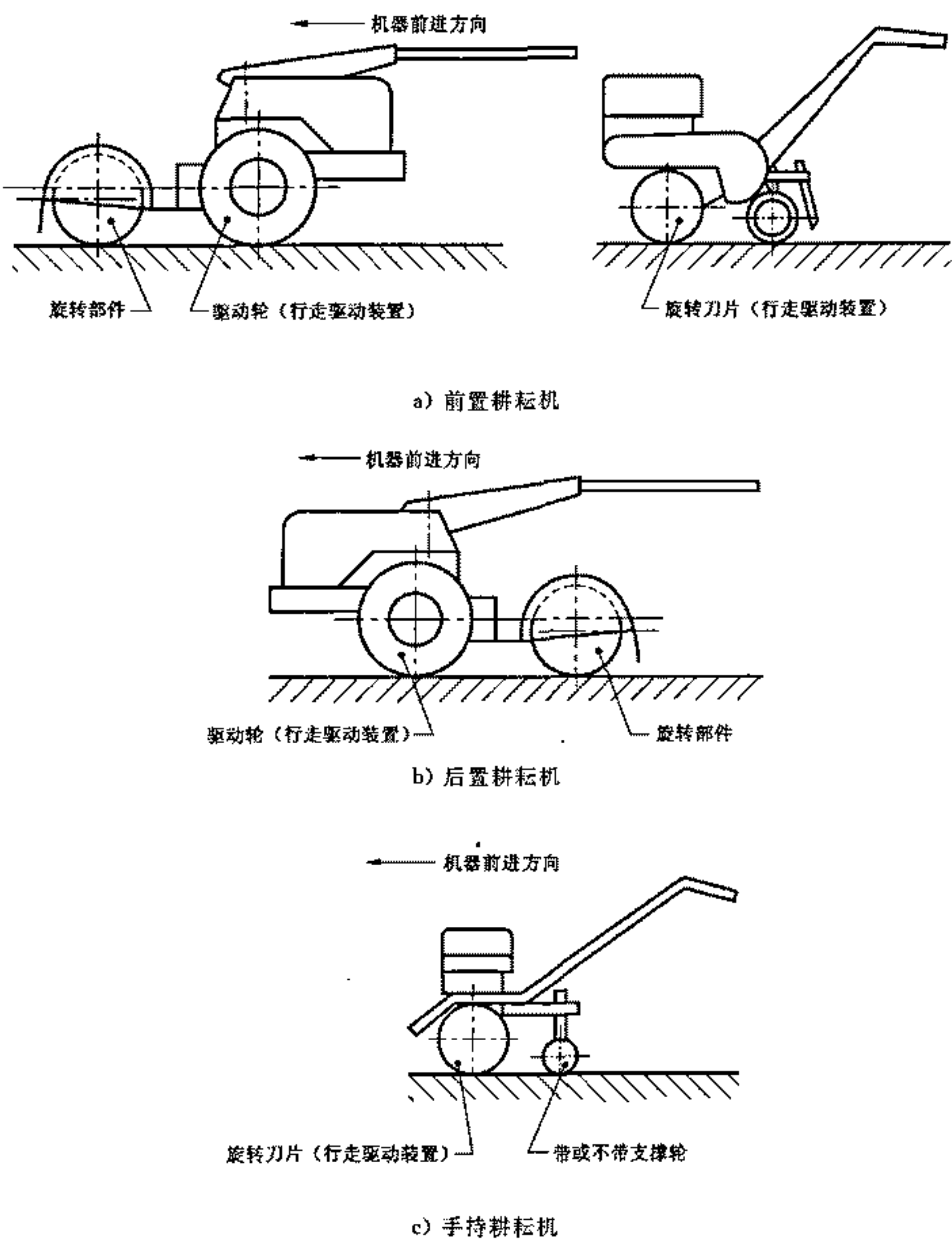
图 1 耕耘机的型式
