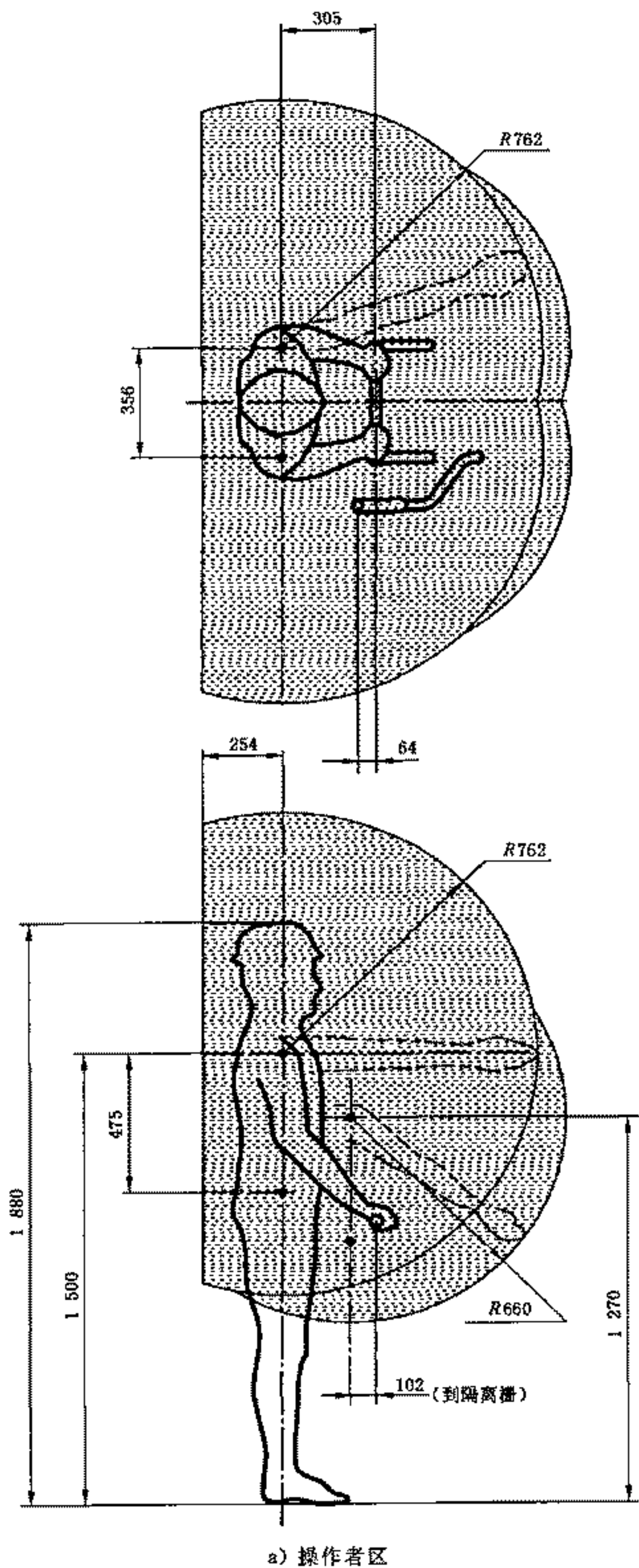
图 5 手扶(步行操纵)机器的操作者区
